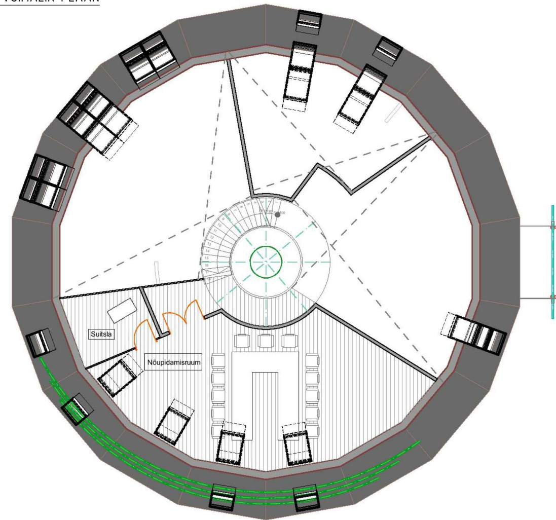
TEISE KORRUSE VÕIMALIK PLAAN
